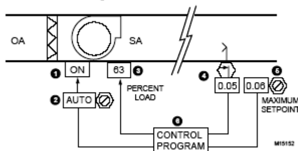
شکل (۱-۵) توصیف عملکردی استفاده از یک هواساز برای تامین هوای تازه چندین هواساز
