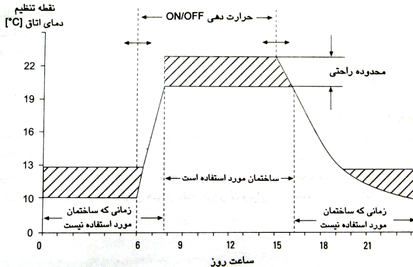
شکل (۱) کلیدزنی متغیر
