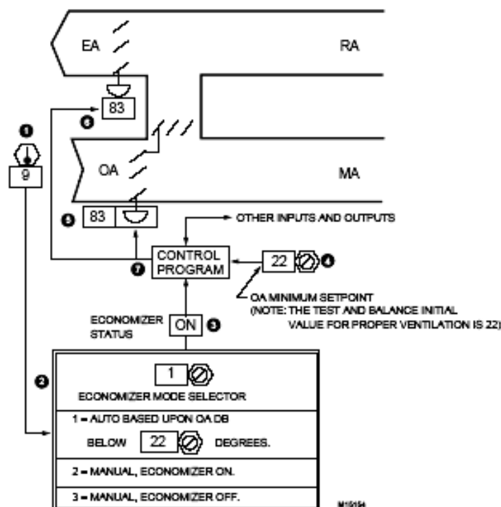
شکل (۱-۱۱) توصیف عملکردی کنترل با توجه به درجه حرارت خشک هوای بیرون
