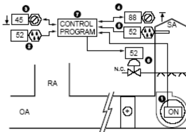
شکل (۱-۲۵) فرآیند رطوبت زنی
