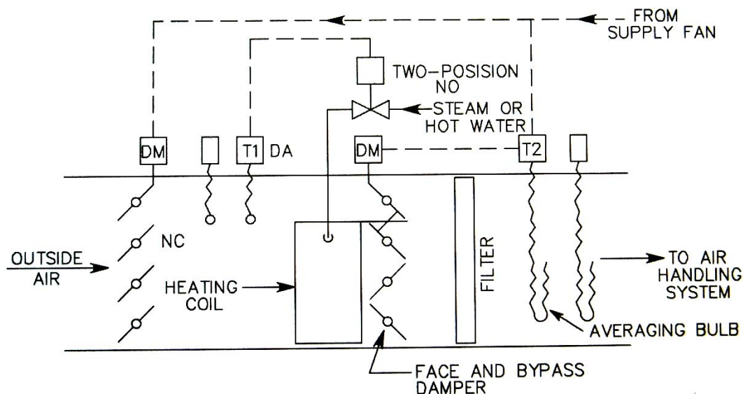
شکل (۲۰-۱) جلوگیری از یخ زدن کویل پیش گرمایش
