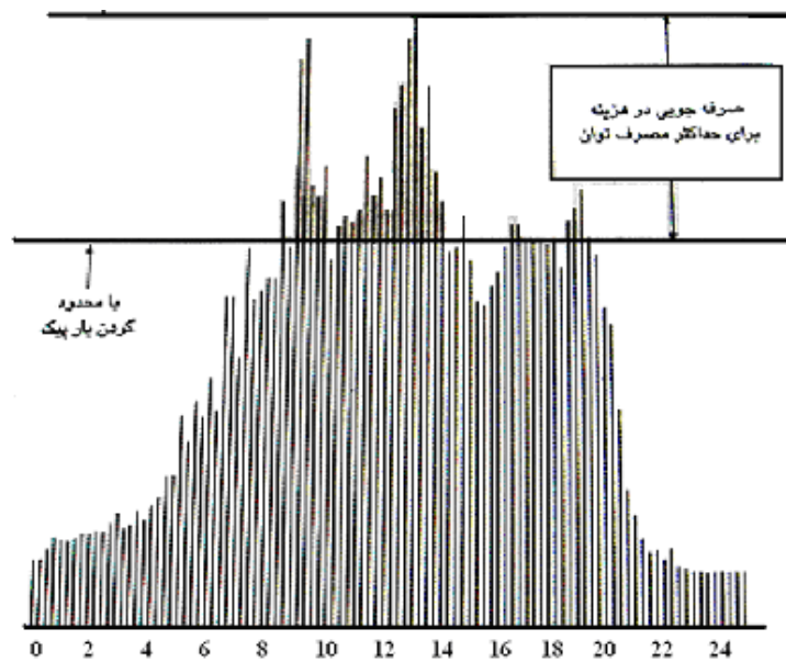
شکل (۳) محدود کردن بار پیک
