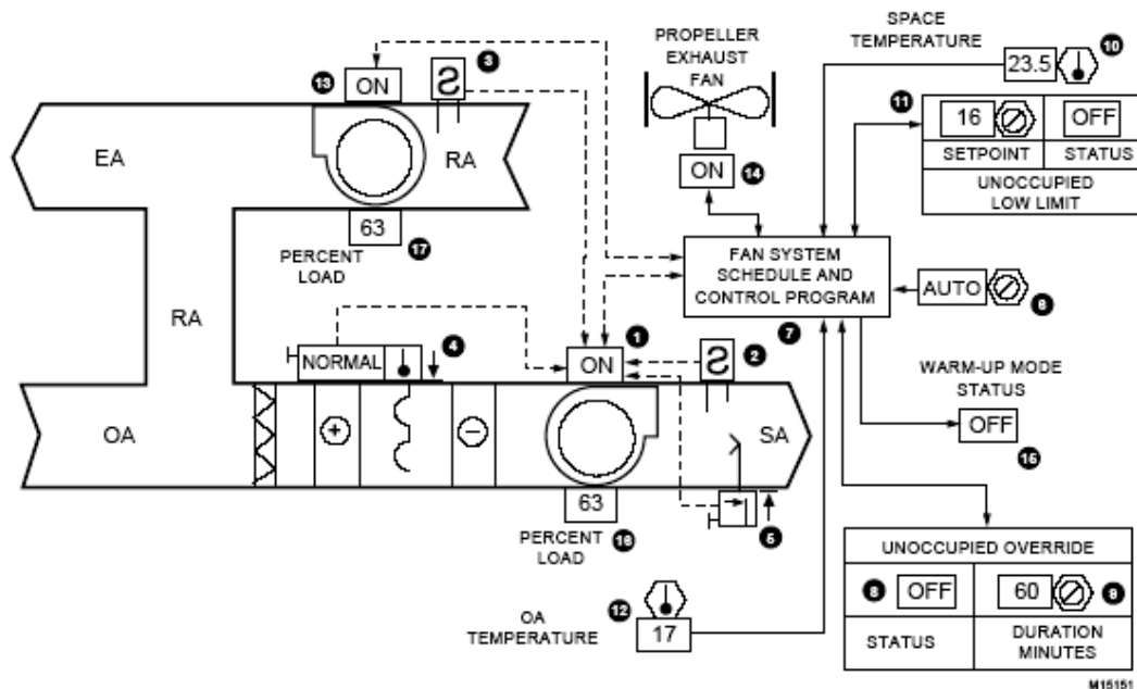
شکل (۱-۱) توصیف عملکردی روشن-خاموش شدن فن هواساز
