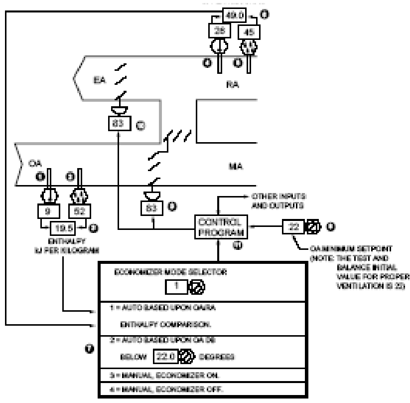
شکل (۱-۱۳) مقایسه انتالپی هوای برگشت و هوای بیرون
