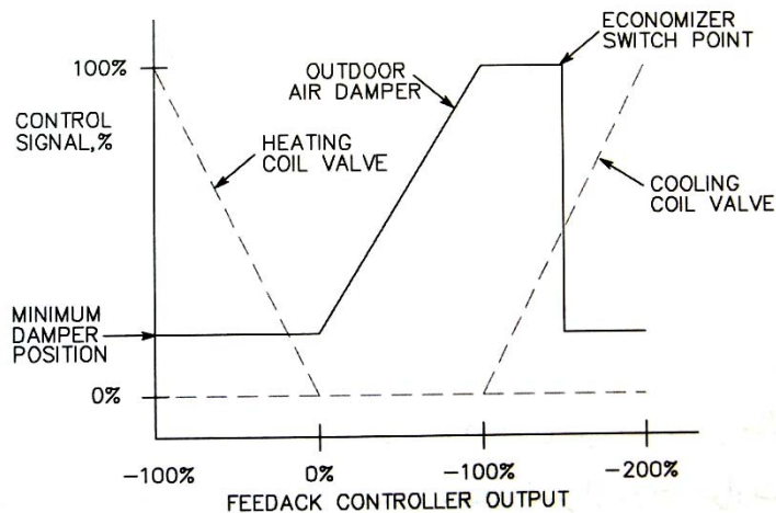
شکل (۹-۱) شرایط مختلف در چرخه با صرفه
