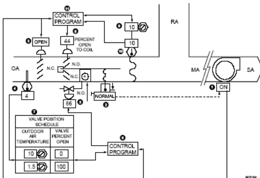
شکل (۱-۲۲) توصیف عملکردی کنترل پیش گرمایش از طریق دمپرهاى رخ و کنارگذر
