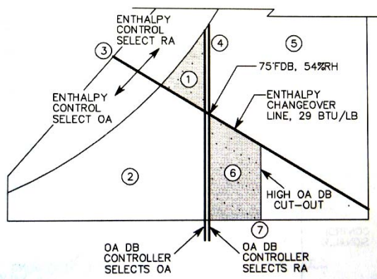
شکل (۱۰-۱) نمودار سایکرومتریک چرخه با صرفه
